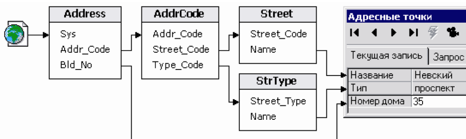
Рисунок 14.1. Схема данных
